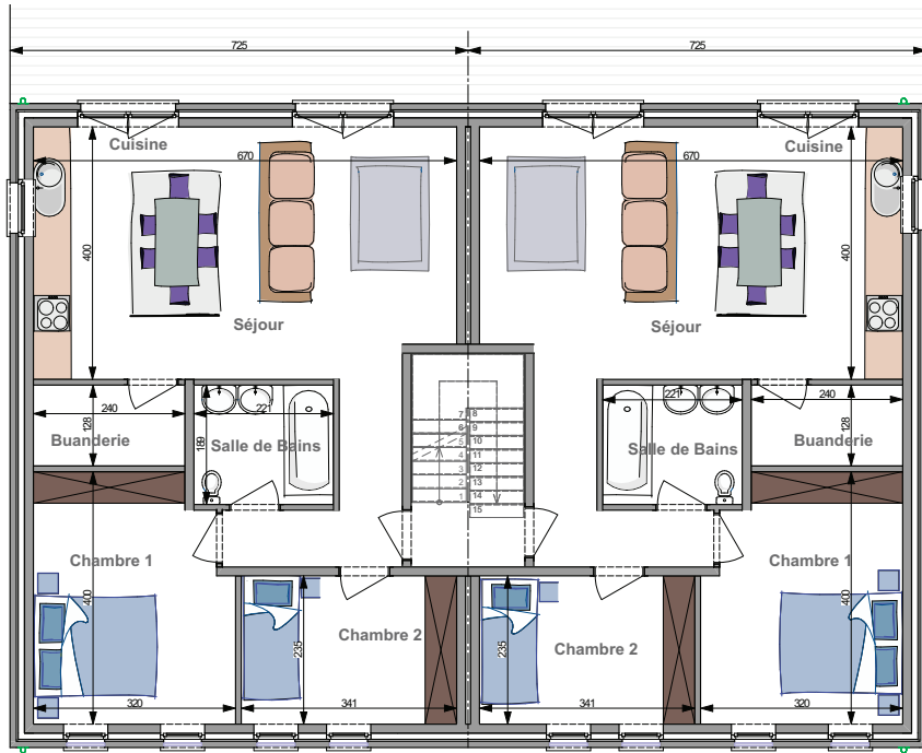
ÉTAGE 1
