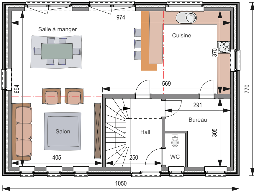
REZ-DE-CHAUSSÉE
